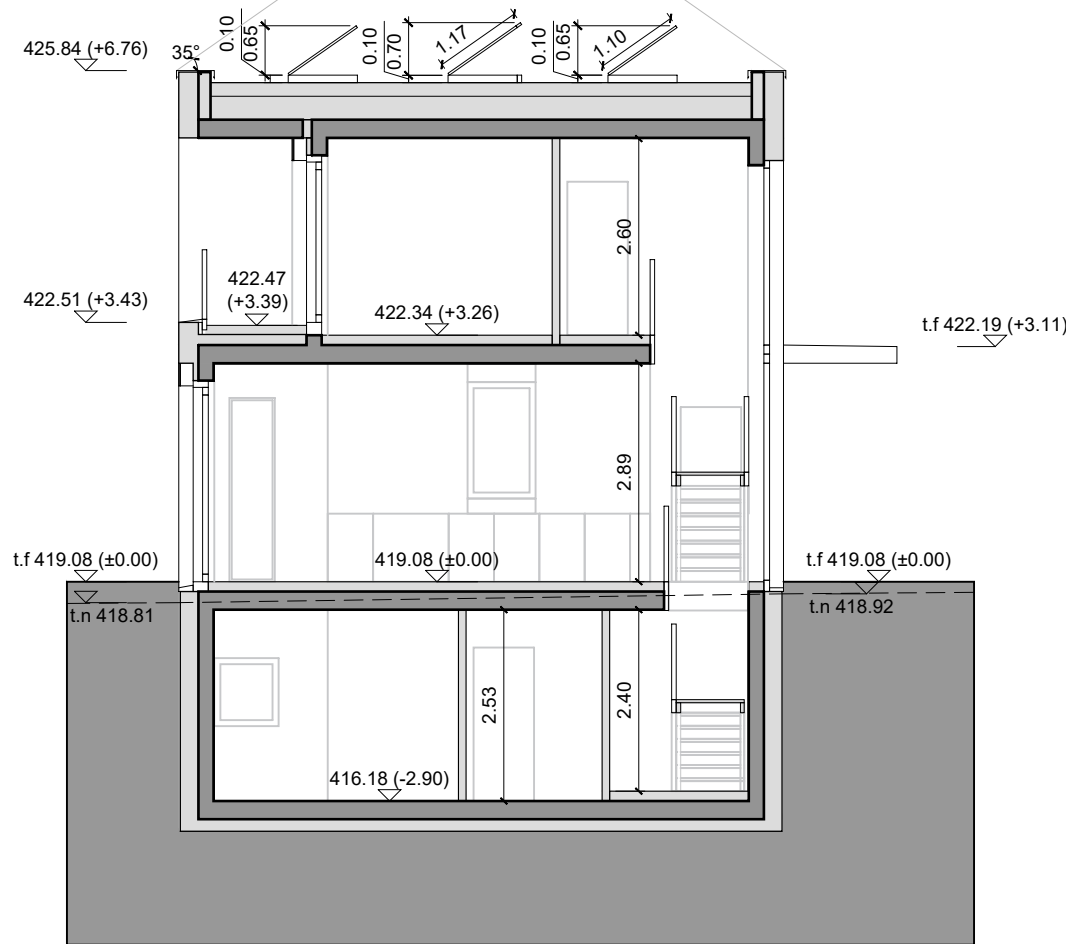
Coupe B-B
